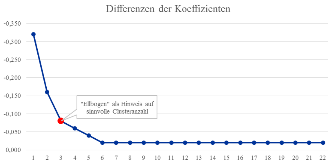
Abbildung 32: Diagramm zur Bestimmung des Elbow-Kriteriums
