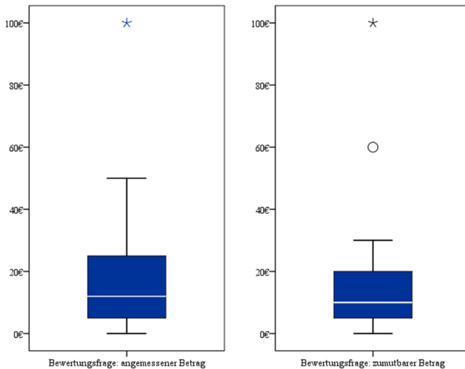
Abbildung 52: Bewertungsfragen: Boxplots
