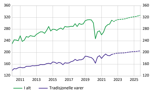
Figur 2.13. Import
