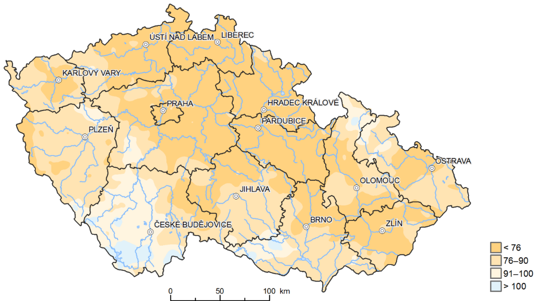
Obr. 3.1.1.9 Úhrn srážek v procentech normálu 1981–2010 v r. 2018
