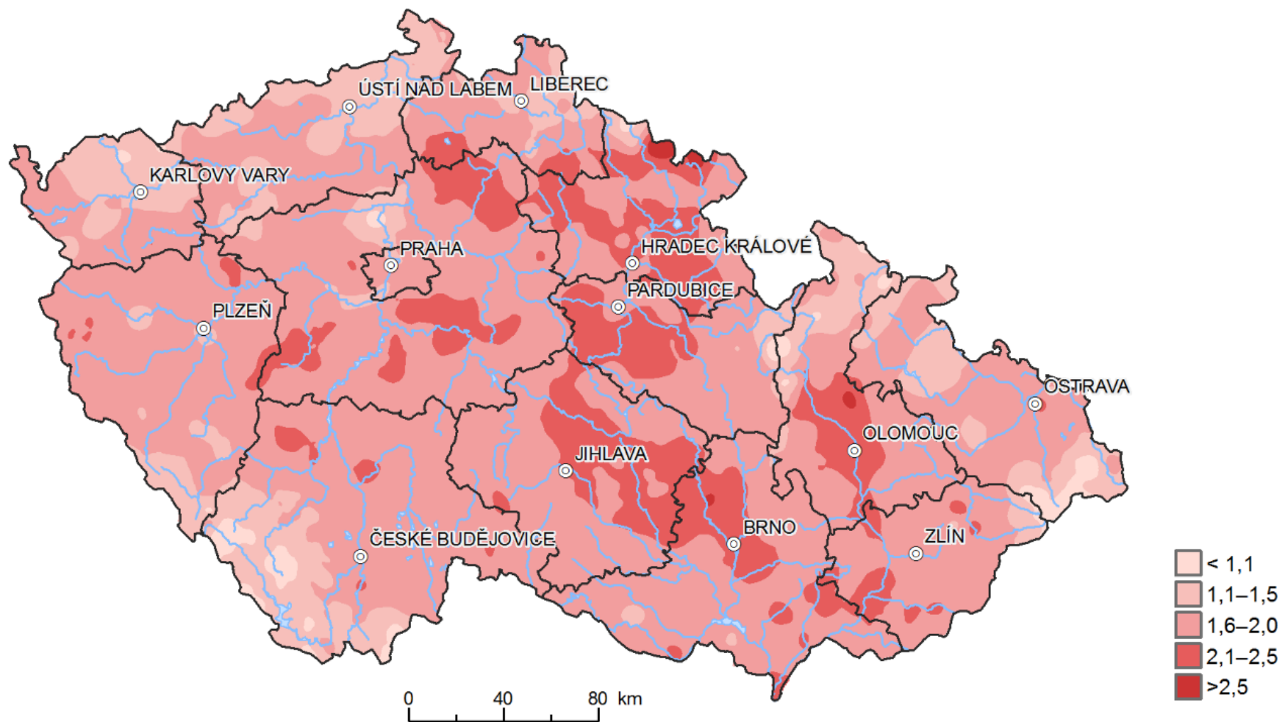
Obr. 3.1.1.7 Odchylka průměrné roční teploty vzduchu od normálu 1981–2010 v r. 2018 [°C]
