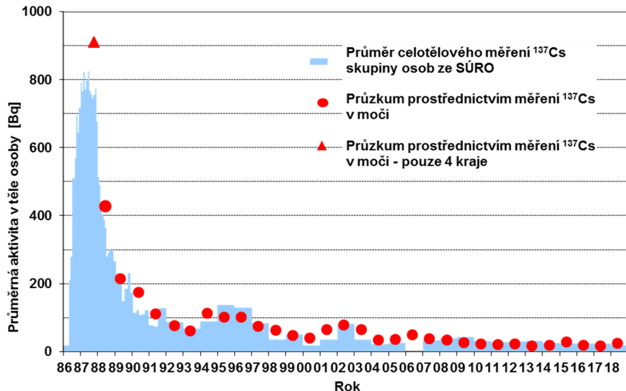
Obr. 3.7.1.1 Vývoj obsahu ^{137}\text{Cs} u českého obyvatelstva po černobylské havárii, 1986–2018
