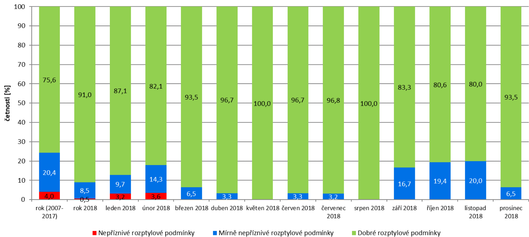
Obr. 3.2.3.1 Roční chod procentuálního výskytu rozptylových podmínek na území ČR v roce 2018
