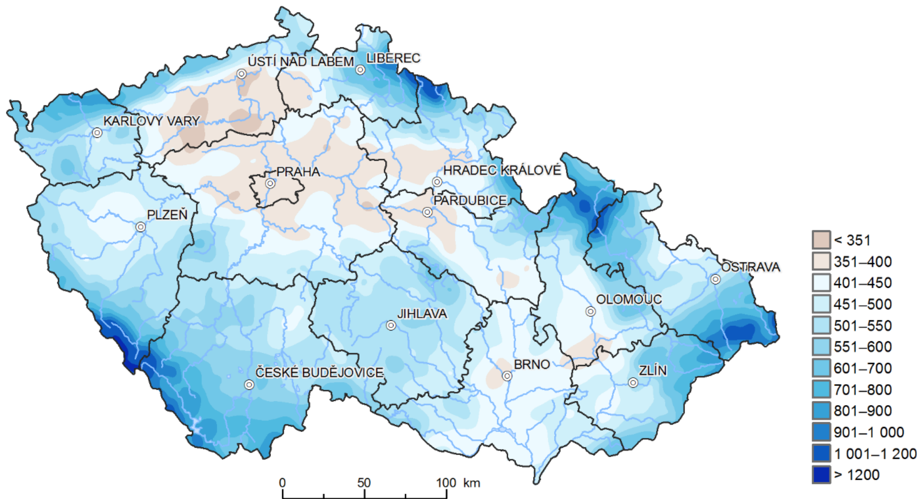
Obr. 3.1.1.8 Roční úhrn srážek v r. 2018 [mm]
