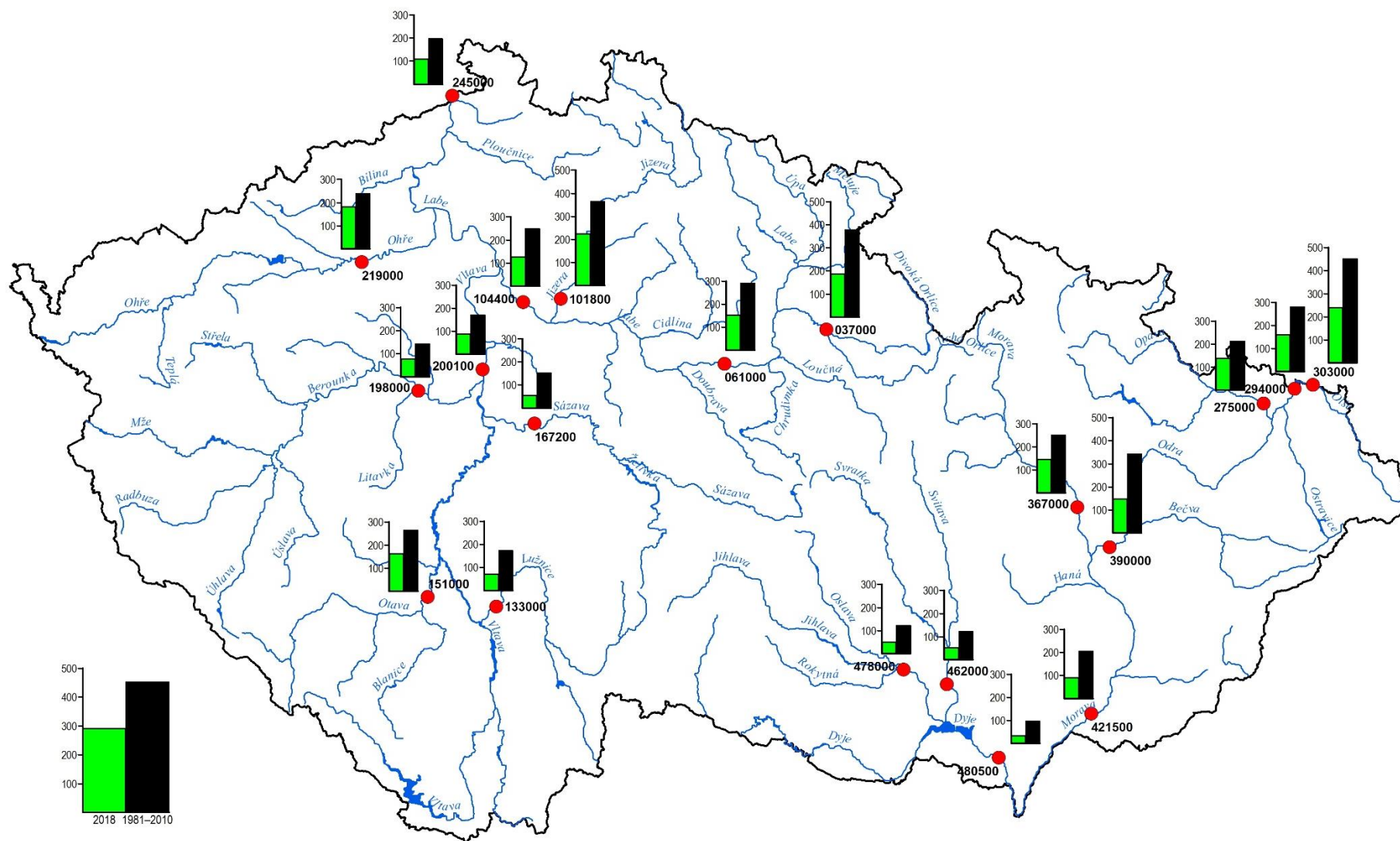
Obr. 3.3.1.3 Odtokové výšky za hydrologický rok 2018 v porovnání s dlouhodobým průměrem, 1981–2010
