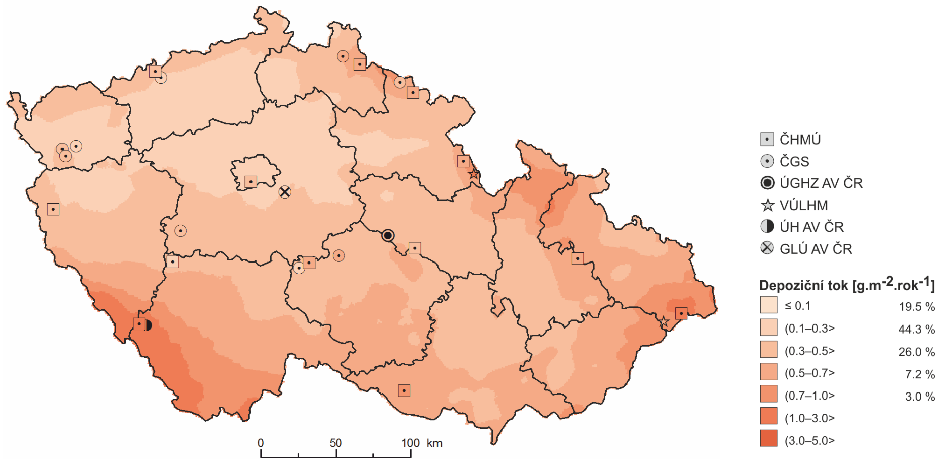
Obr. 3.2.2.18 Pole mokré roční depozice olovnatých iontů, 2018
